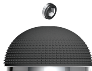
Plasmafit® Plus ohne Bohrungen, mit Verschlusskappe
